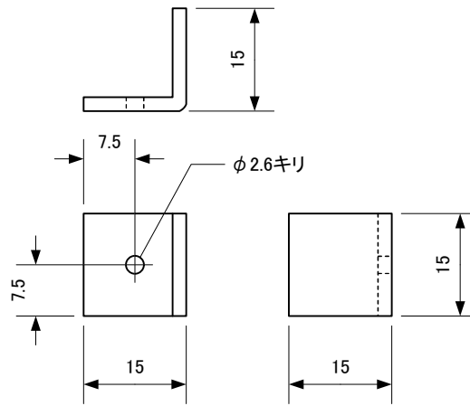
固定板(4個)
