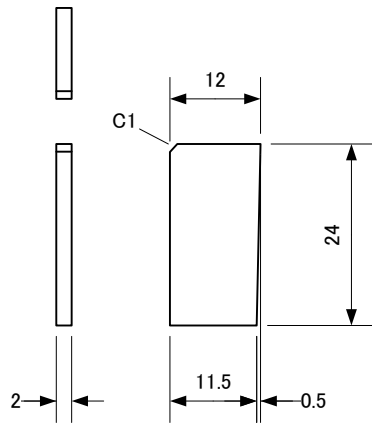
補強板(1個)
